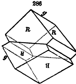
Calcite.
